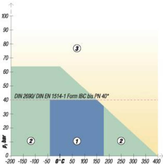
Gráfico Presión x Temperatura
